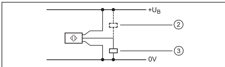
Abb. 6: Dreileitertechnik
