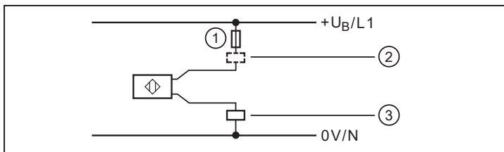
Abb. 5: Zweileitertechnik
